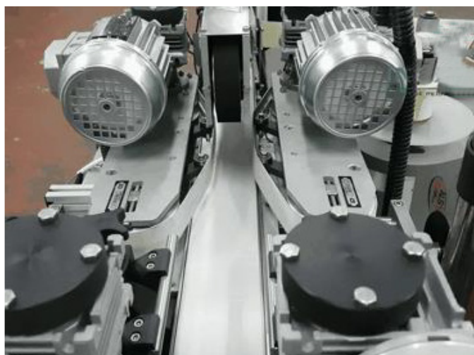
Узел выравнивания тары на конвейерной ленте привод протяжной ленты
