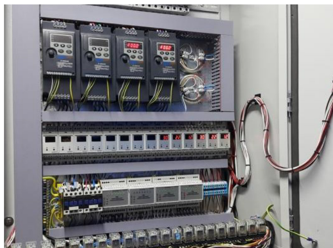
Шкаф управления
